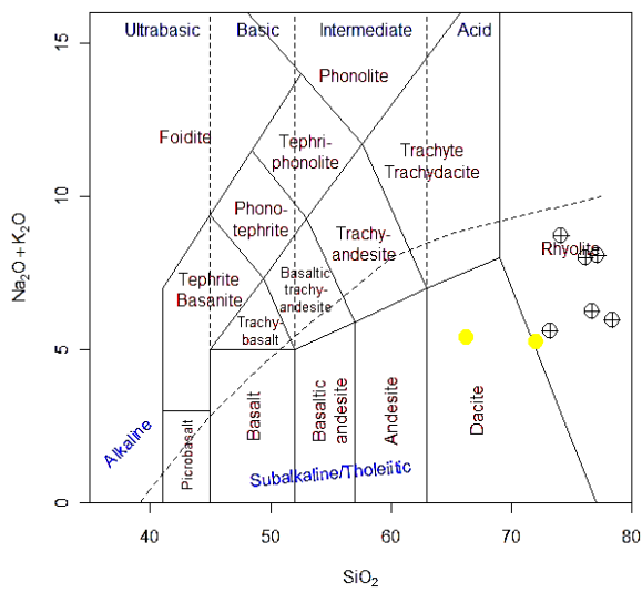
Fig. 6. Classification of rhyolite rocks (Le Bas et al , 1986).
